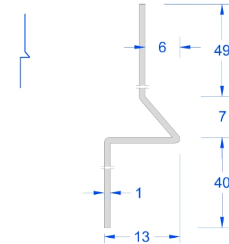
maxit Dachbelüftungsprofil
